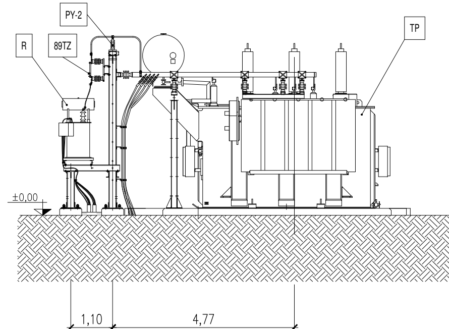
SECCIÓN B-B
