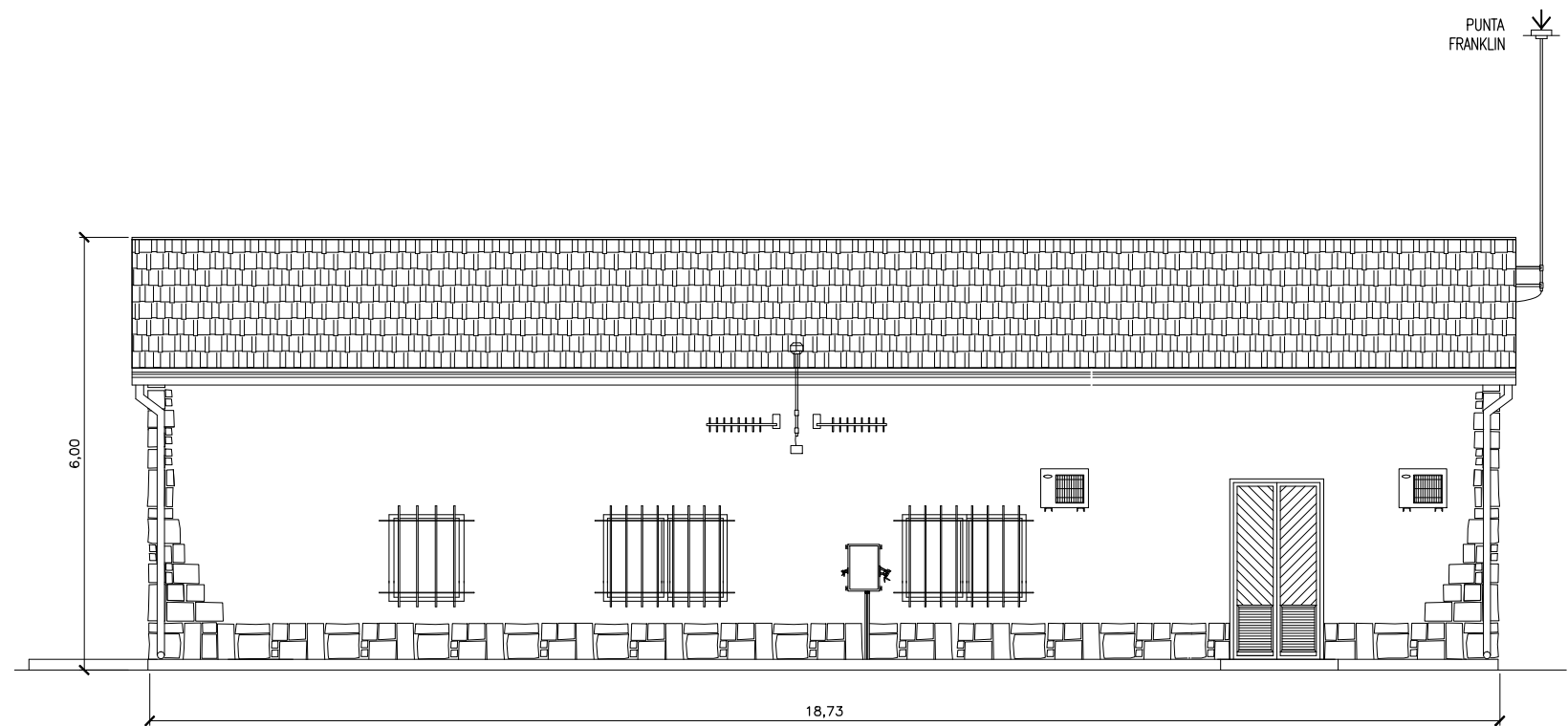
FACHADA POSTERIOR
